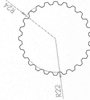
Presek ozubljenе осовине hidрауличне пумпе
